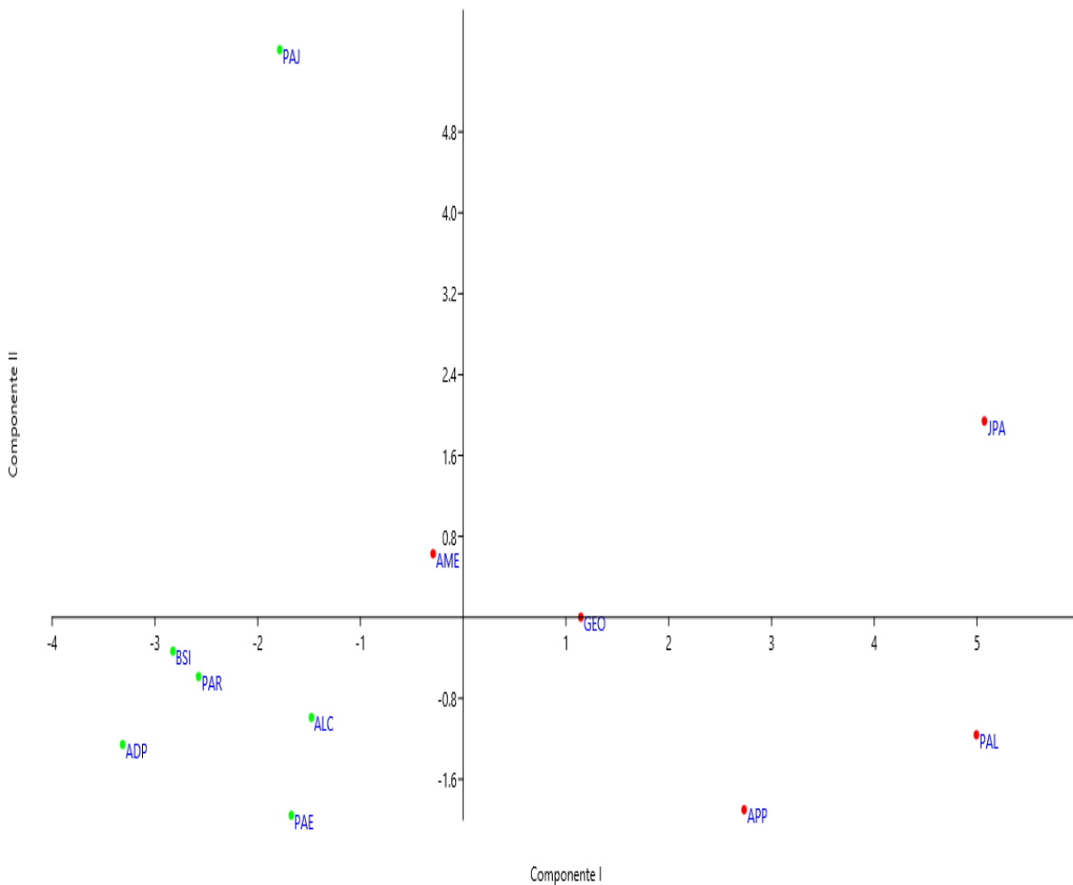
Figura 2. ACP que muestra las relaciones de similitud entre las 11 revistas analizadas. % de la varianza acumulada: 93,83. Para los acrónimos, véase Metodología.
