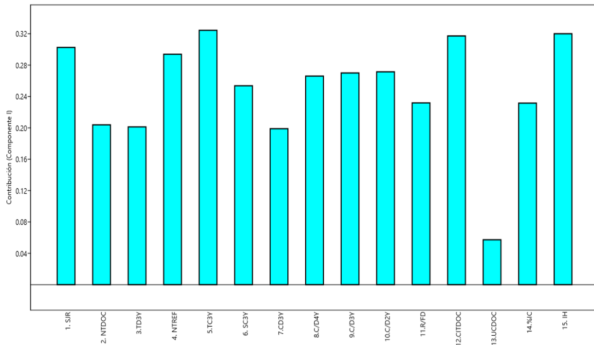
Figura 3. Gráfico que muestra la contribución de los 15 indicadores al componente principal I. Para los acrónimos, véase Metodología.
