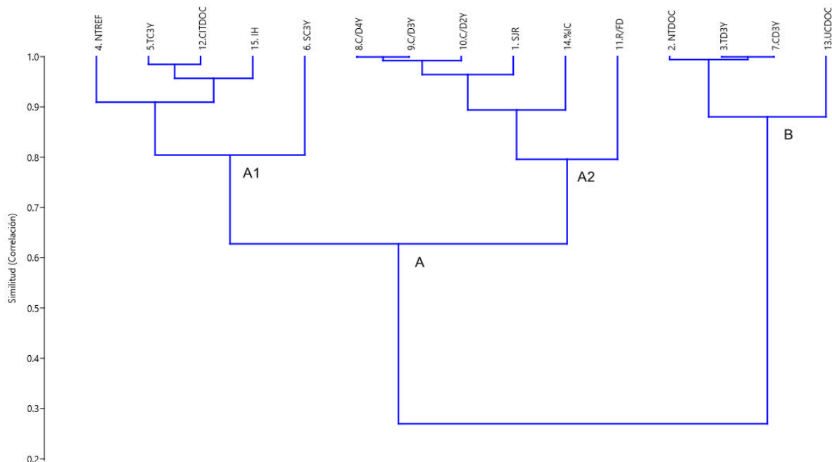
Figura 1. Fenograma (UPGMA) que muestra las relaciones de similitud (correlación) entre los 15 indicadores considerados. CCC: 0,718. Referencias: A y B: grupos; A1 y A2: subgrupos. Para los acrónimos, véase Metodología.
